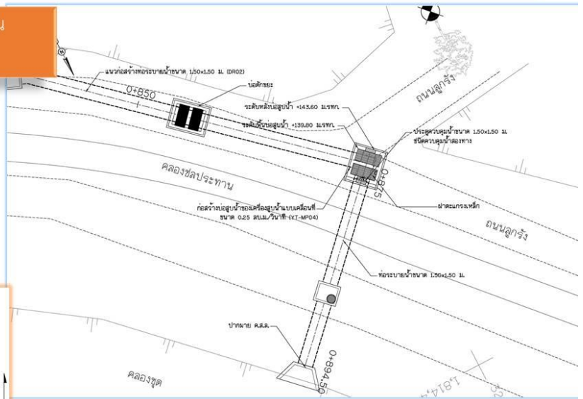
MP04 บ่อสูบน้ำ บริเวณปลายท่อระบายน้ำ DR02
